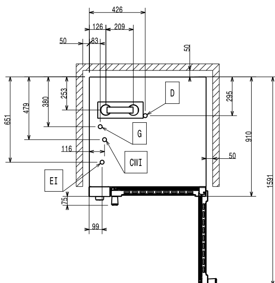
Boven aanzicht
